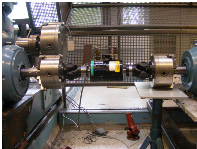
Figur 2.2. Momentmåler
