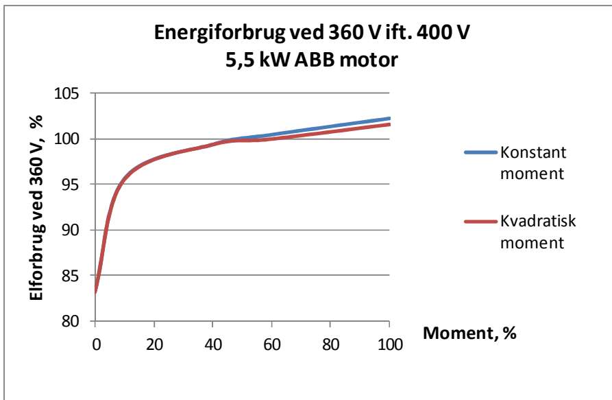
Figur 5.3 Elforbrug ved 360 V ift. elforbruget ved 400V til løsning af konkret opgave
