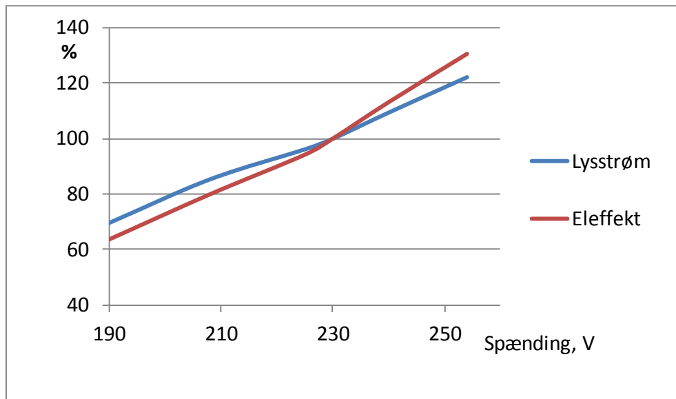
Figur 2. 36 W lysstofrørs optagne elfekt og lysstrøm som funktion af forsyningsspændingen. Armaturet har induktiv spole.
